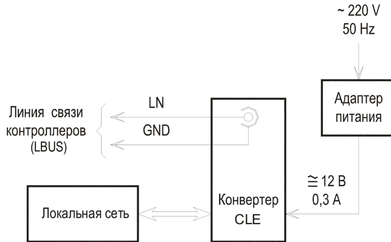
Рис.1. Схема подключения конвертера CLE
